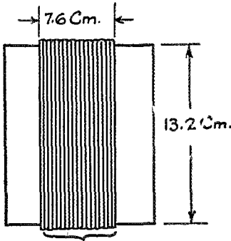
53 turns 20 D.C.C.
